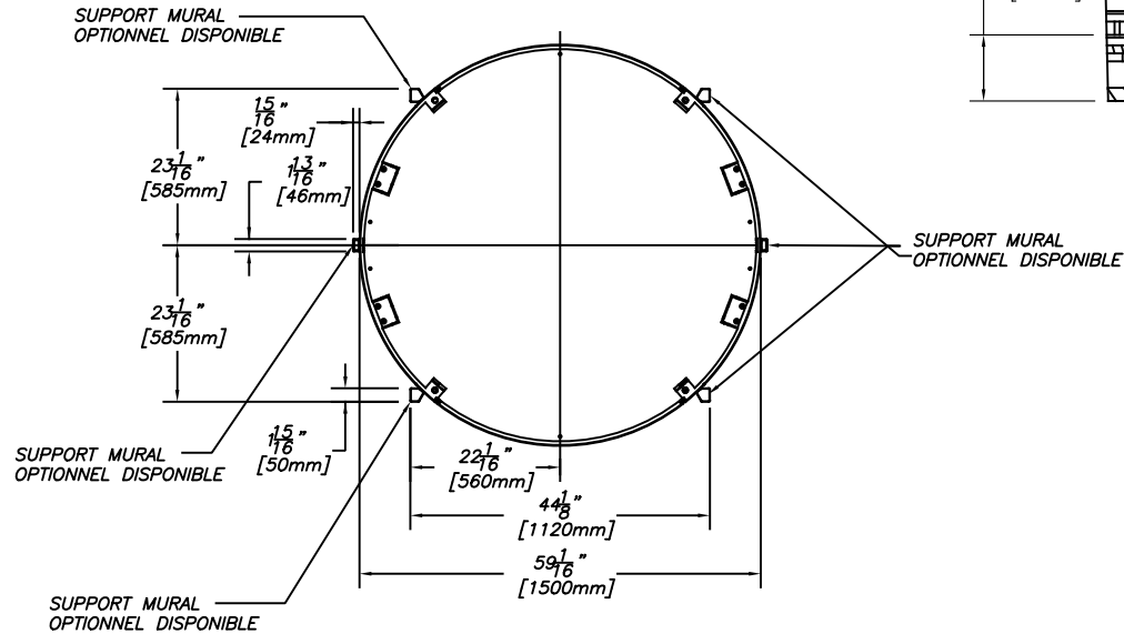
VUE DE COUPE B-B
