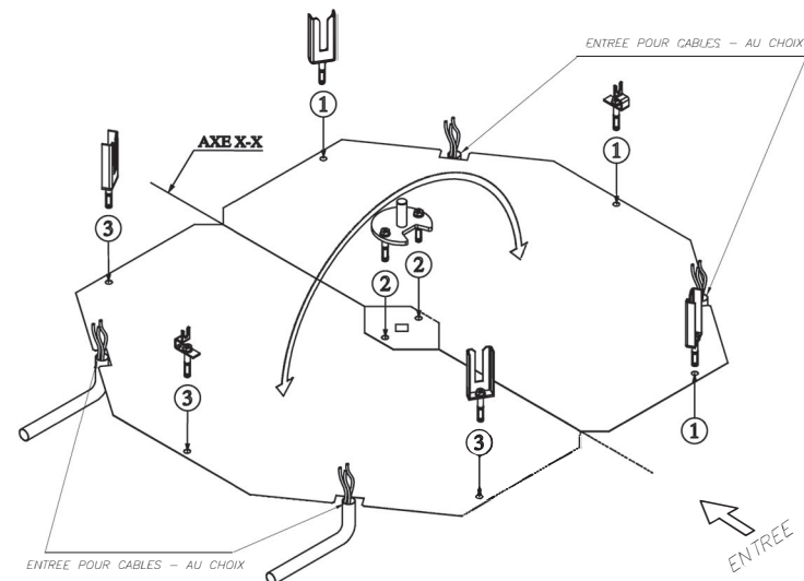
POSITIONNEMENT DU GABARIT – ITEM NO. GAB-E-0007770
